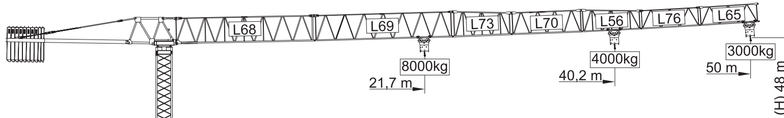
Cargas.Loads.Lasten.Charges.Cargas.Carichi.Yükler. ГРУЗОПОДЪЁМНОСТЬ
